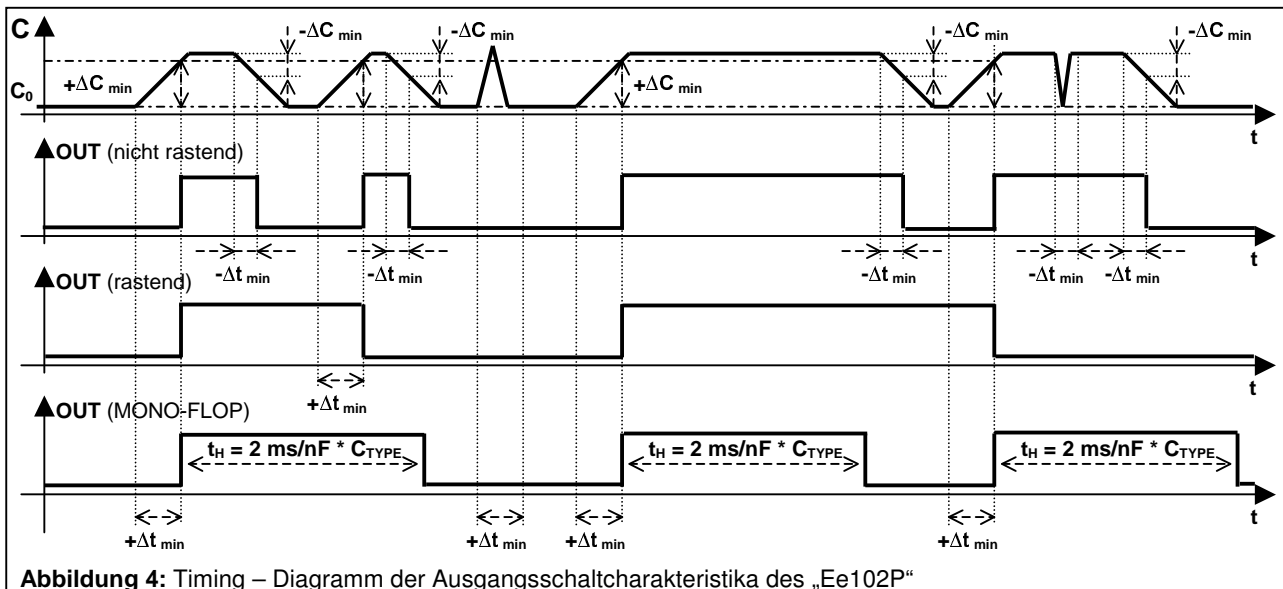
Abbildung 4: Timing – Diagramm der Ausgangsschaltcharakteristika des „Ee102P“
